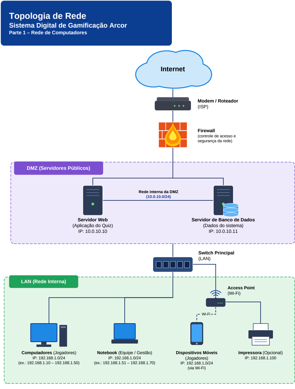
Figura 1 – Topologia de rede do Sistema Digital de Gamificação Arcor (diagrama elaborado no Draw.io).
